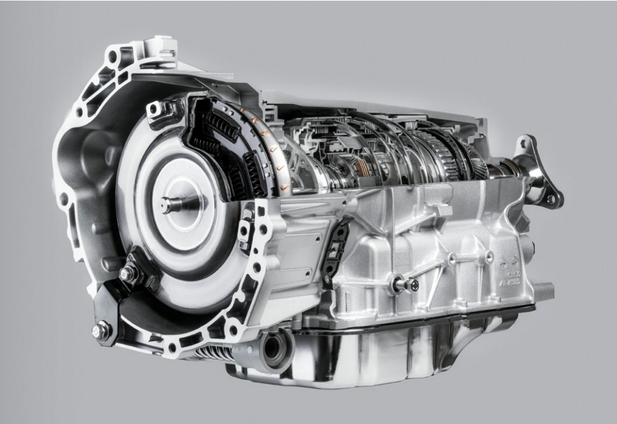
Powerglide 6L50 de fabricación de PUNCH Powerglide Strasbourg
